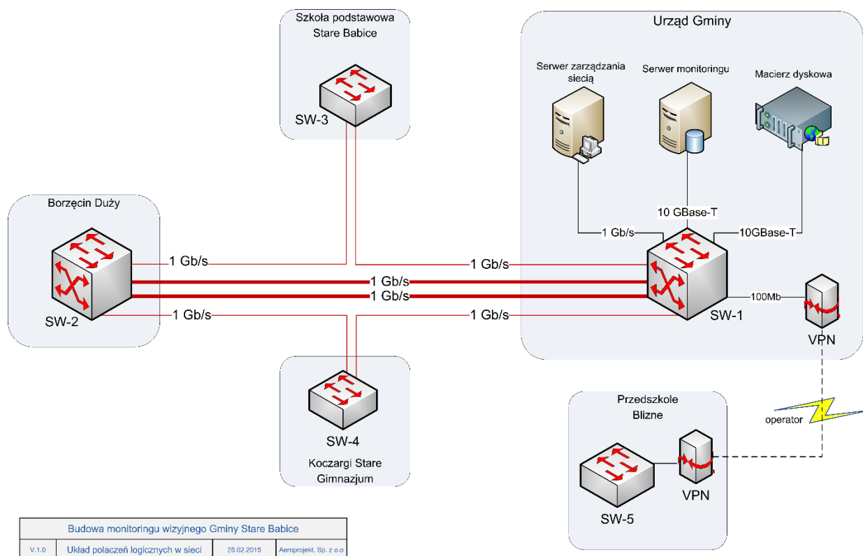
Rysunek 60 - schemat połączeń logicznych sieci
