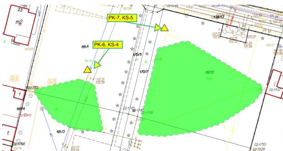
Rysunek 15 - KS-4 - obszar obserwacji kamery
