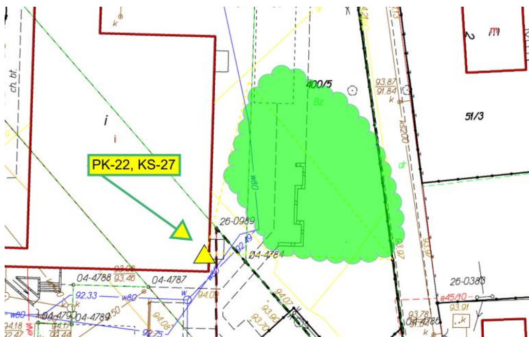
Rysunek 46 - KS-27 - propozycja umieszczenia kamery
