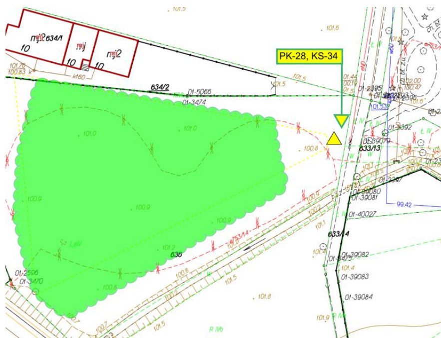
Rysunek 59 - KS-34 - obszar obserwacji kamery
